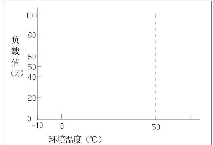
输出负载降额与环境温度关系
